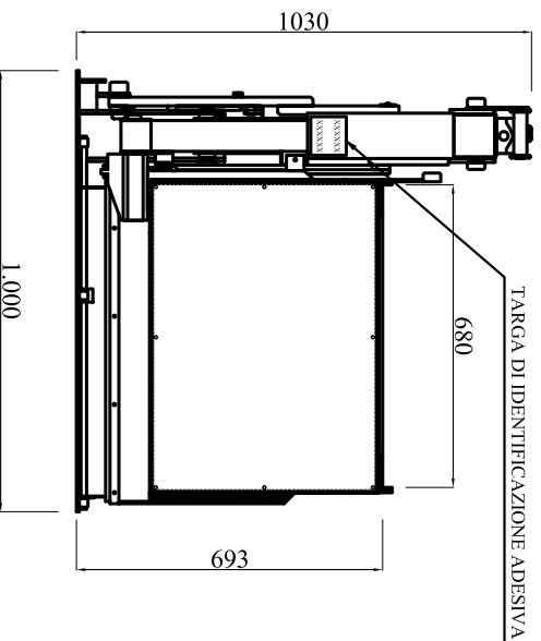
VISTA FRONTALE SOLLEVATORE
