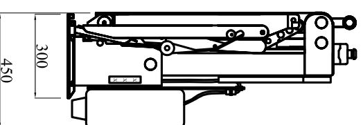
VISTA LATERALE DEL SOLLEVATORE CHIUSO
